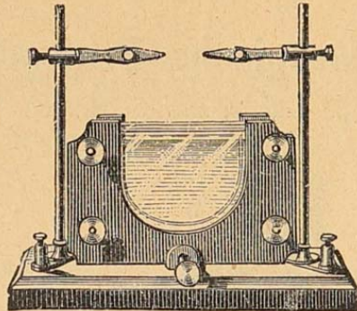
Electrische Cüvette.
