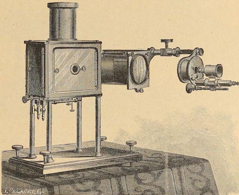
Universitäts-Projections-Apparat mit Polariscope in Verbindung mit Microscop.
